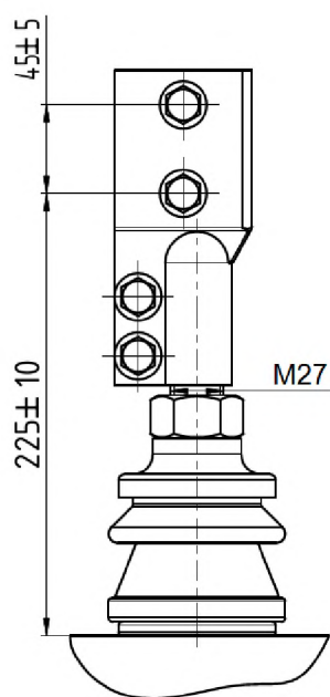
Рисунок А.5 – Ввод НН на номинальный ток 1000 А
