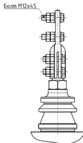
Рисунок А.5 – Ввод НН на номинальный ток 1000 А
