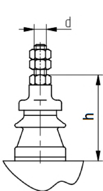
Рисунок А.4 – Ввод НН на номинальные токи до 630 А
