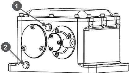
Рис. 20 Замена масла в вибраторе
