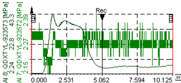
Рисунок 7 – Показатели электросистемы
