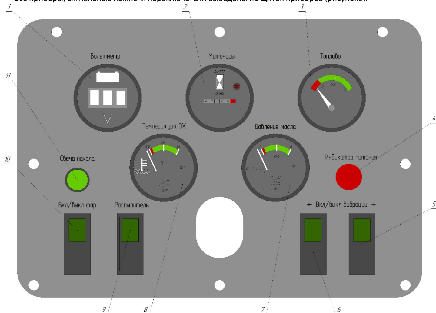
Рисунок 9 – Щиток приборов
