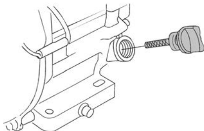
Рис. 8 Крышка-щуп маслосливной горловины
