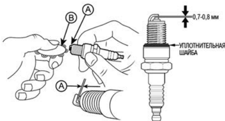
Рис. 23 Проверка зазора между электродами
