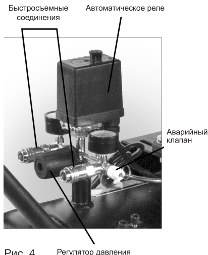
Рис. 4 Регулятор давления
