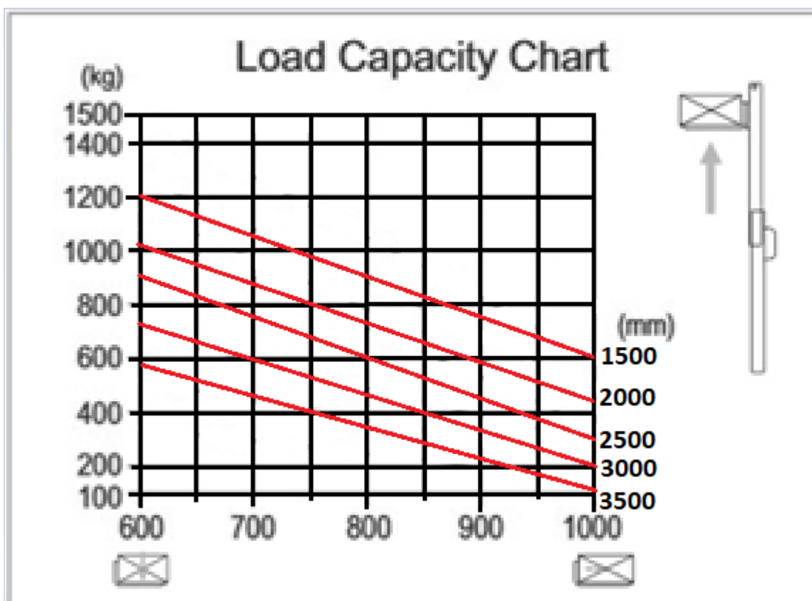
График грузоподъемности
