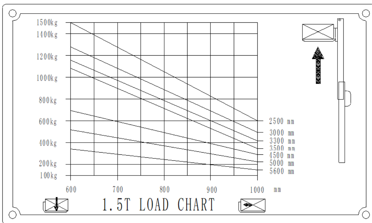
Рис.2 - График грузоподъемности
