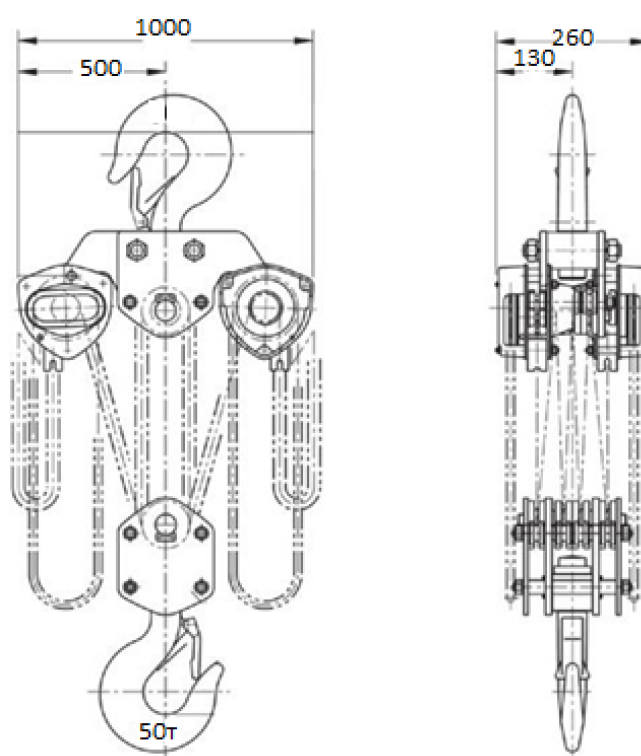
Рис. 1- Основные размеры тали
