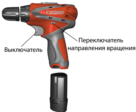
Рисунок 5. Переключатель направления
