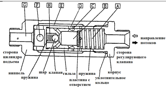
клапан регулятора расхода
