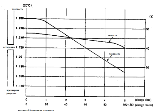
рисунок 6-3 зависимость плотности
