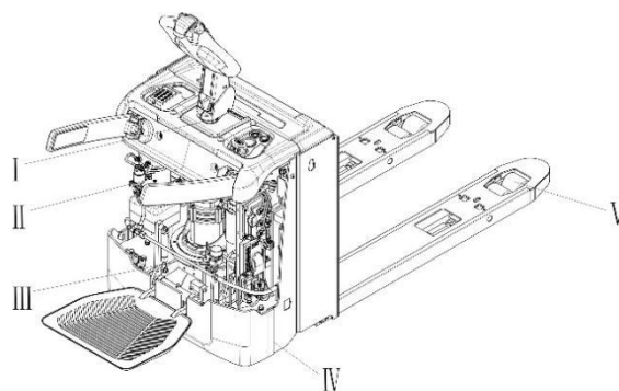
Рис. 14: Точки смазки
