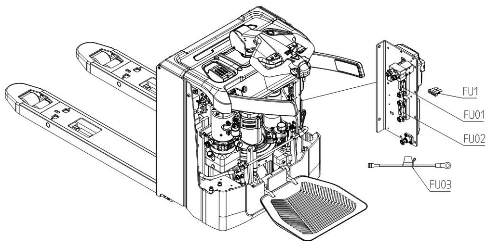
Рис. 15: Расположение предохранителей
