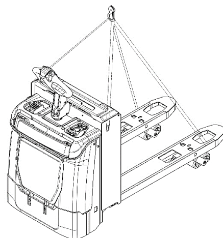
Рис. 5: Подъем краном
