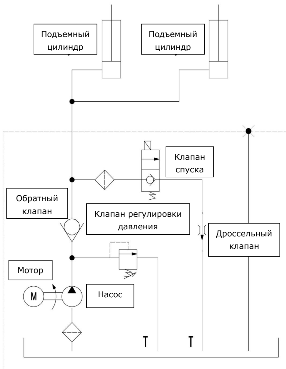
Рис. 17: Гидравлическая схема
