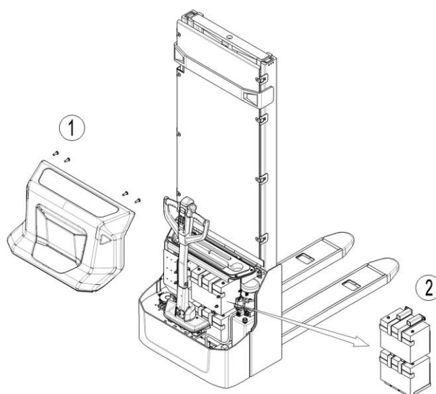
Рис. 12: Замена АКБ
