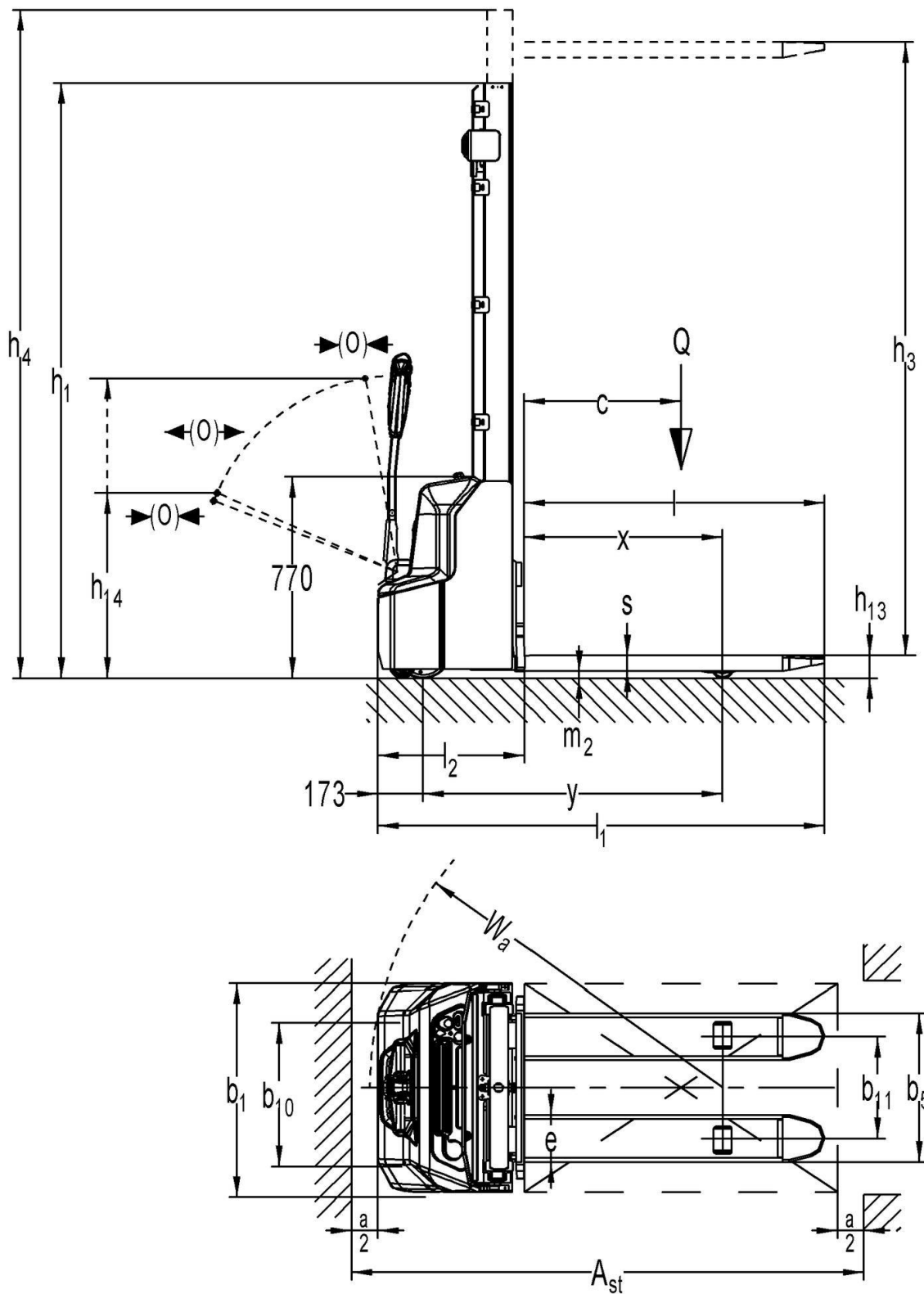
Рис. 2: Технические характеристики
