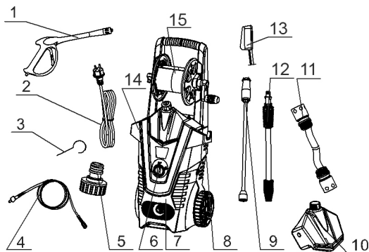
Рисунок 1 – Устройство изделия
