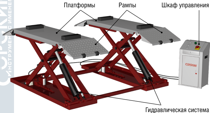
Рисунок 1 – Комплект поставки
