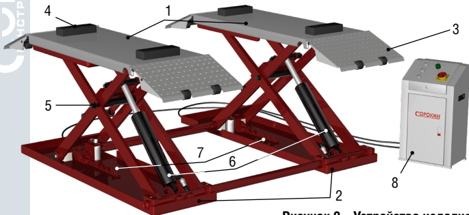
Рисунок 2 – Устройство изделия
