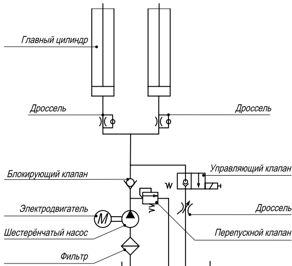
Рисунок 6 – Гидравлическая схема
