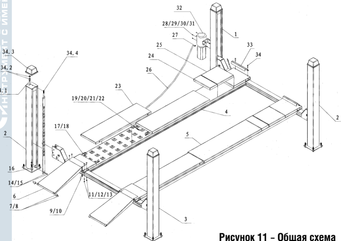
Рисунок 11 – Общая схема
