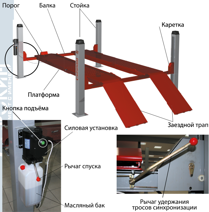
Рисунок 2 – Устройство изделия
