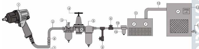
Рисунок 5 – Пневматическая схема подключения
