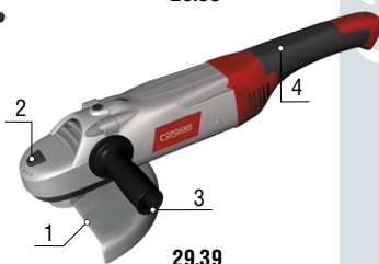
Рисунок 1 - Устройство изделия
