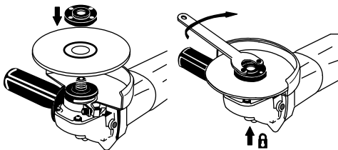
Рисунок 2 – Установка диска
